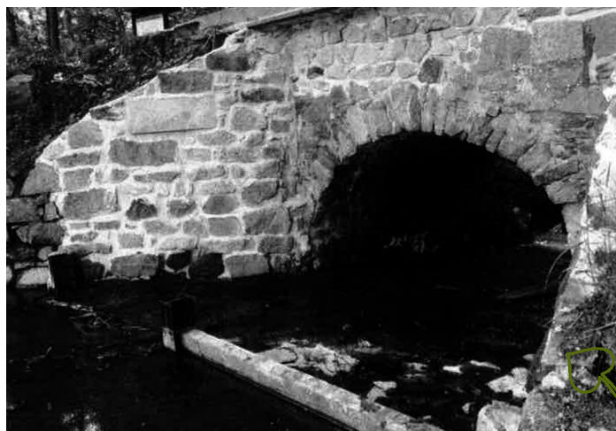
Můstek nad bezpečnostním přelivem Struhařovského rybníka na podzim 2013 a v zimě po opravě.
